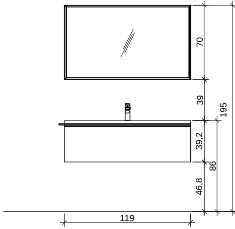
ÖN GÖRÜNÜŞ
