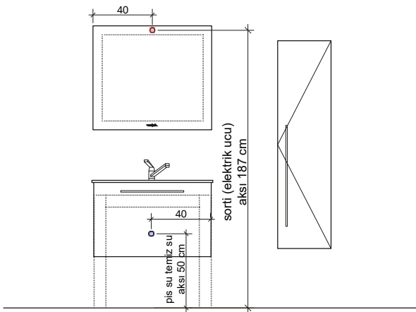
ÖN GÖRÜNÜŞ
