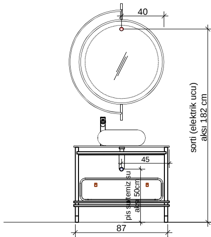
ÖN GÖRÜNÜŞ
