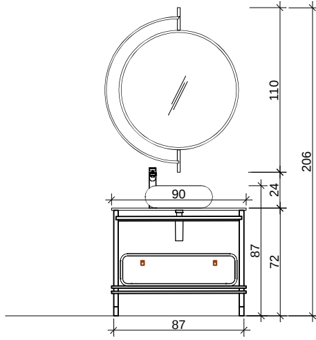
ÖN GÖRÜNÜŞ
