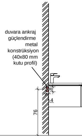
YAN GÖRÜNÜŞ
