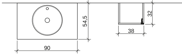
PLAN GÖRÜNÜŞ
