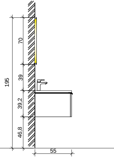
YAN GÖRÜNÜŞ
