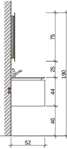
YAN GÖRÜNÜŞ
