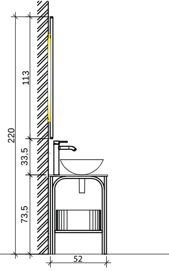
YAN GÖRÜNÜŞ
