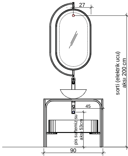
ÖN GÖRÜNÜŞ
