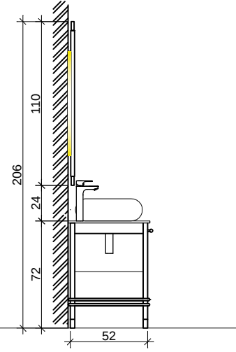
YAN GÖRÜNÜŞ
