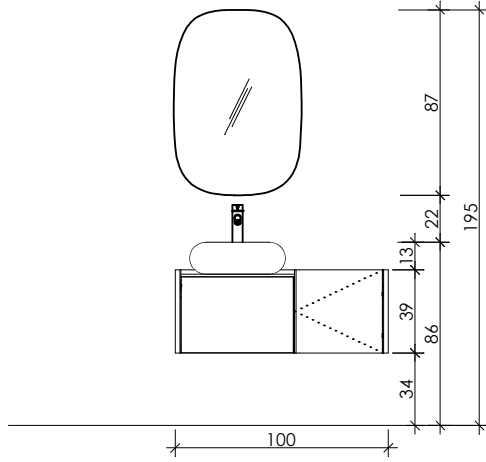
ÖN GÖRÜNÜŞ
