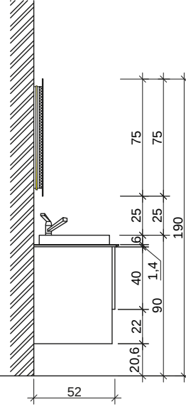
YAN GÖRÜNÜŞ
