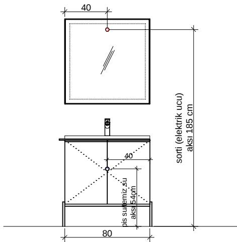
ÖN GÖRÜNÜŞ
