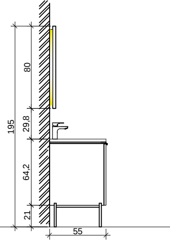
YAN GÖRÜNÜŞ
