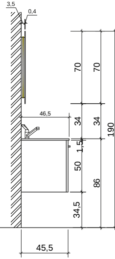
YAN GÖRÜNÜŞ
