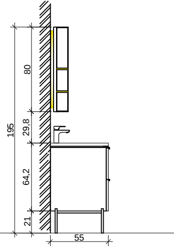
YAN GÖRÜNÜŞ
