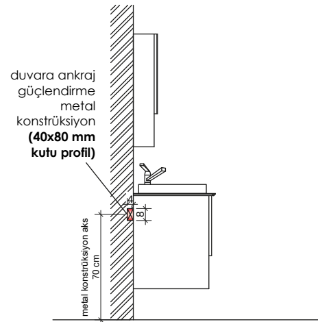
YAN GÖRÜNÜŞ
