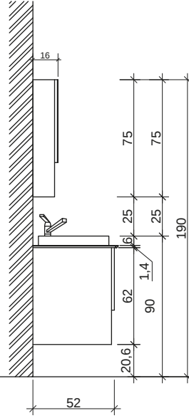
YAN GÖRÜNÜŞ
