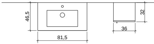
PLAN GÖRÜNÜŞ
