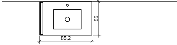
PLAN GÖRÜNÜŞ
