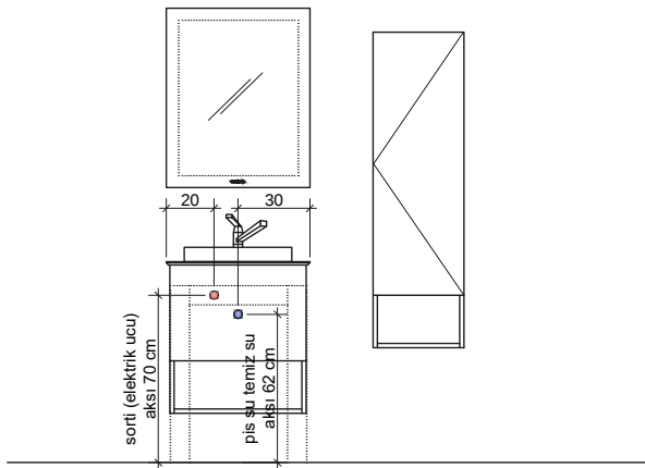
ÖN GÖRÜNÜŞ
