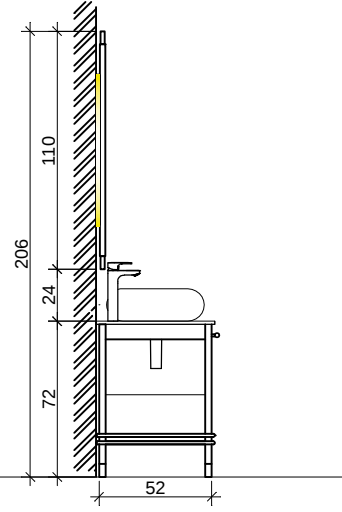
YAN GÖRÜNÜŞ
