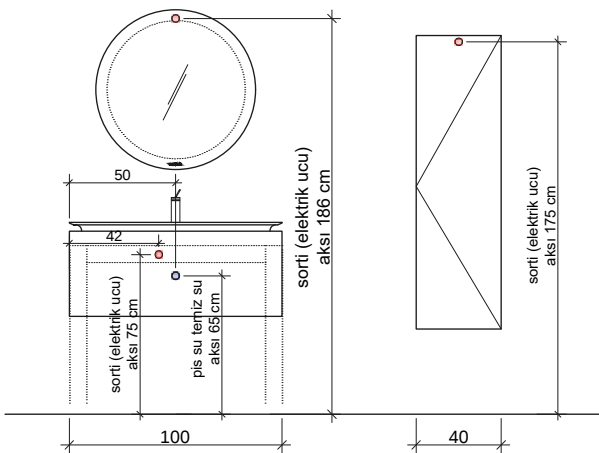
ÖN GÖRÜNÜŞ
