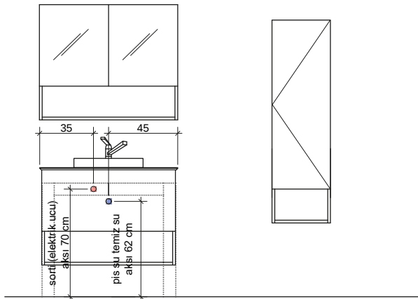
ÖN GÖRÜNÜŞ
