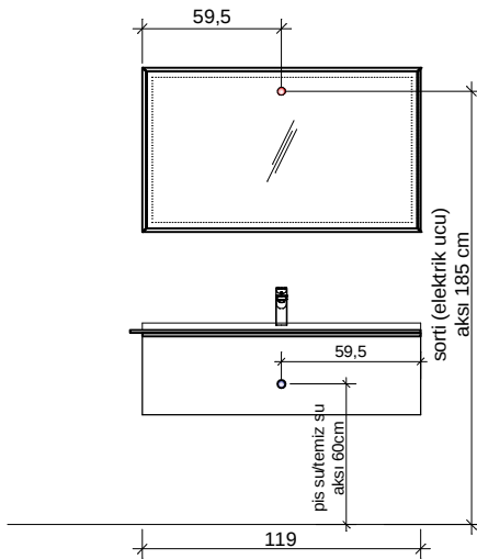
ÖN GÖRÜNÜŞ
