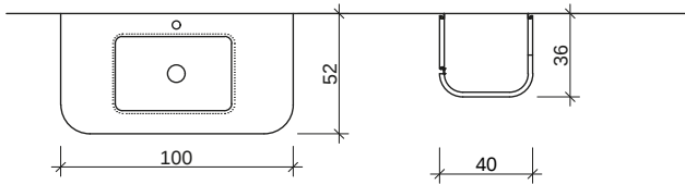
PLAN GÖRÜNÜŞ
