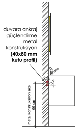
YAN GÖRÜNÜŞ
