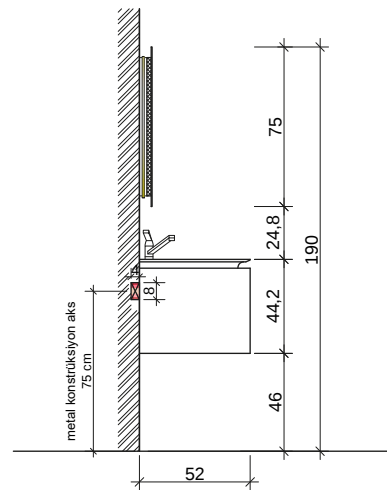
YAN GÖRÜNÜŞ
