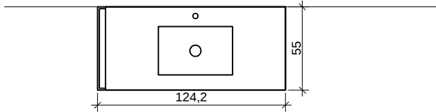
PLAN GÖRÜNÜŞ
