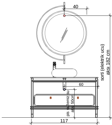
ÖN GÖRÜNÜŞ
