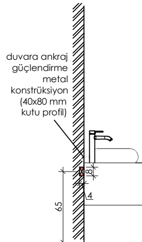
YAN GÖRÜNÜŞ
