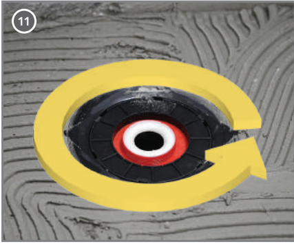
Sifon içerisinde bulunan eksantrik parça ayarı yapılır. Adjust the eccentric part in siphon.
